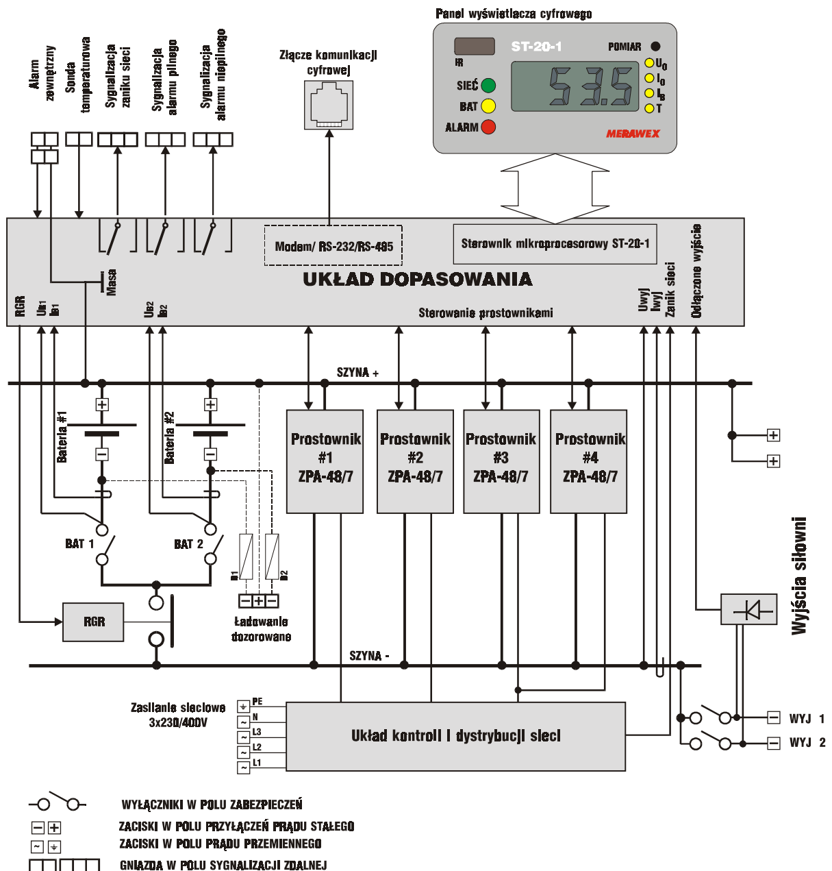
Rys. 3. Schemat blokowy siłowni SI48-28-41
