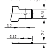
Końcówki biegunowe
