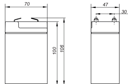
Końcówki biegunowe
